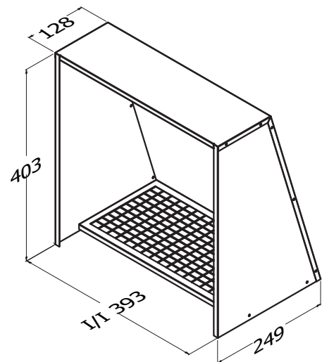
230 WVC 300°
