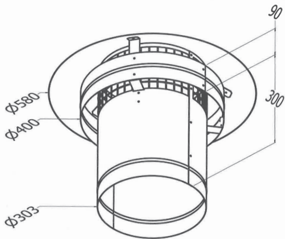
226 DR-300/90°
