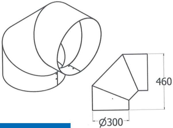
226 DR-300/90°
